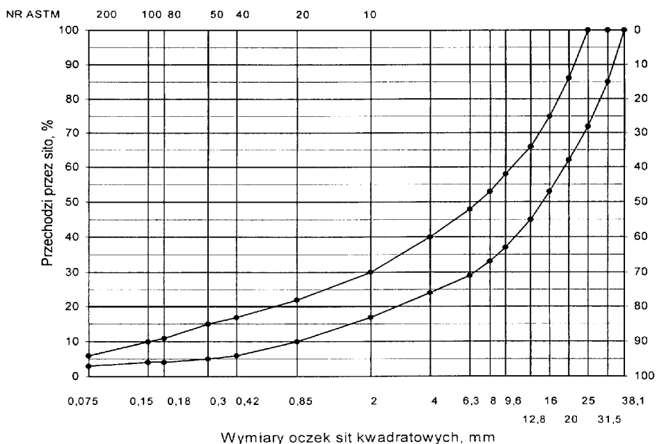
Rys. 6. Krzywe graniczne uziarnieni a mieszanki mineralnej BA od 0 do 31,5 mm podbudow y nawierzch ni drogi o obciążeni u ruchem KR 1 lub KR 2
